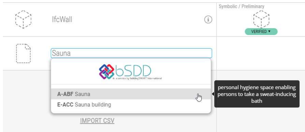
Abb. 3.61: Die Benutzeroberfläche von Plannerly ermöglicht das Durchsuchen des bSDD-Inhalts bei der Erstellung von IDS
