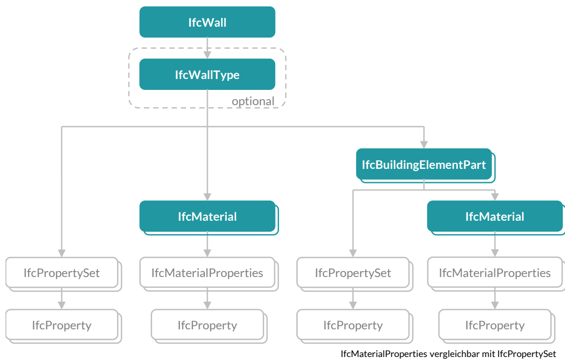
Abb. 3.37: Möglichkeiten von IfcProperty bei einem IfcElement
