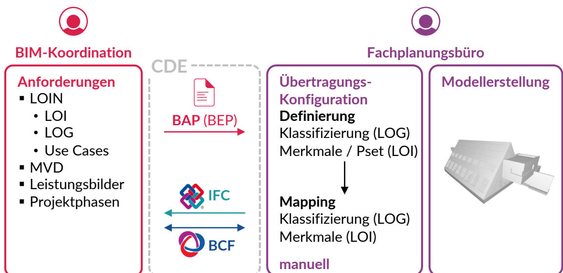
Abb. 3.1: Manuelle Verwaltung von Merkmalen und Klassifizierungen
