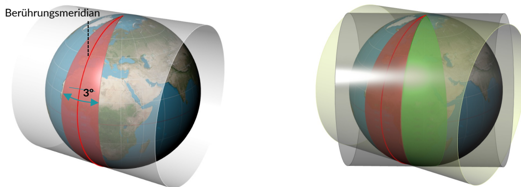
Abb. 3.71: Projektion im GK-System: 3 °-Streifenbreite (links) und Drehung des Projektionszylinders (rechts)
