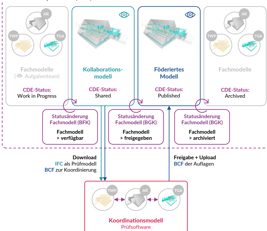
Abb. 4.8: Zusammenhang der Modelltypen mit der CDE und dem BIM-Qualitätsmanagement
