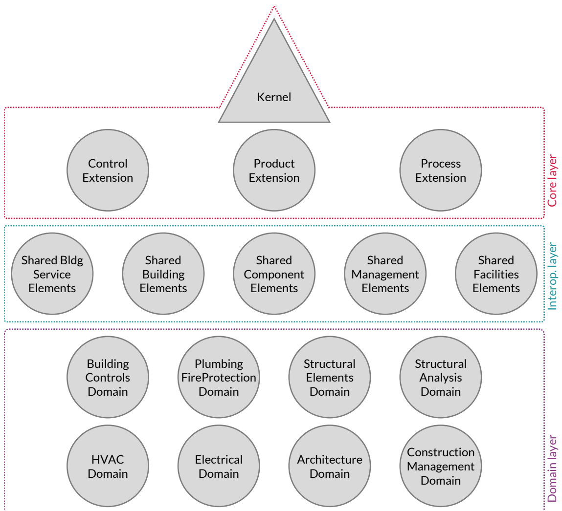
Abb. 3.13: Darstellung der Layerstruktur
