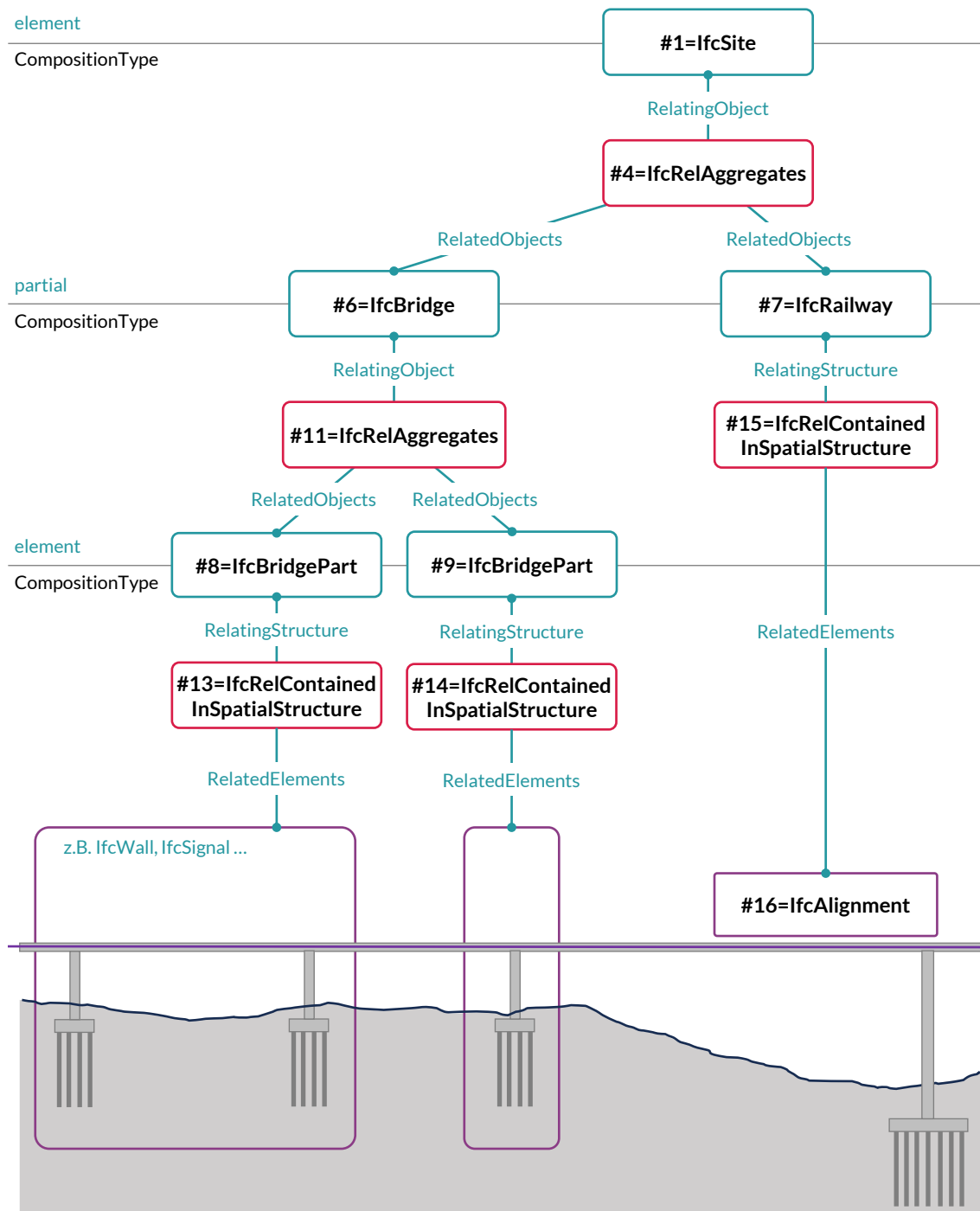
Abb. 3.32: Räumliche Beziehung von Linienbauwerken
