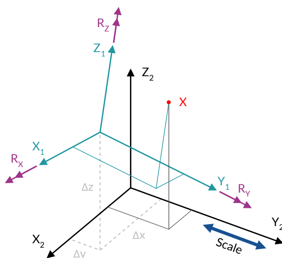
Abb. 3.74: 7-Parameter-Helmert-Transformation (adaptiert von wikimedia, s. QR-Code)
