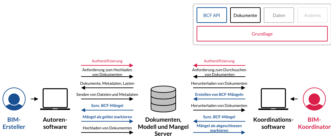
Abb. 3.46: openCDE-Kommunikation BIM-Ersteller und BIM-Koordination
