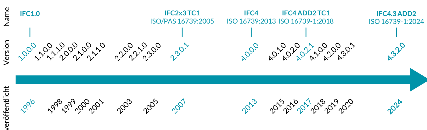
Abb. 3.10: IFC-Versionen
