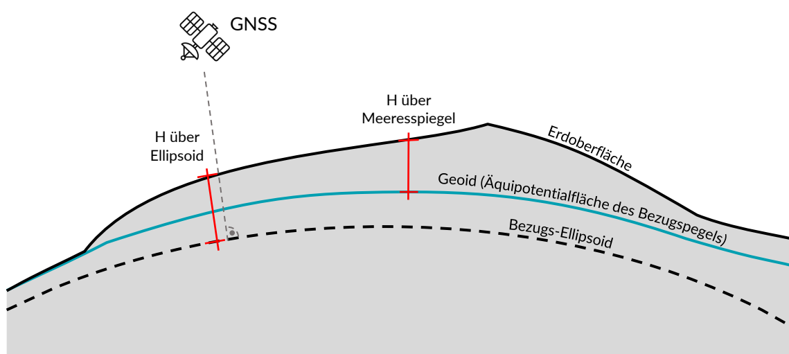
Abb. 3.76: Ellipsoid, Geoid und Erdoberfläche
