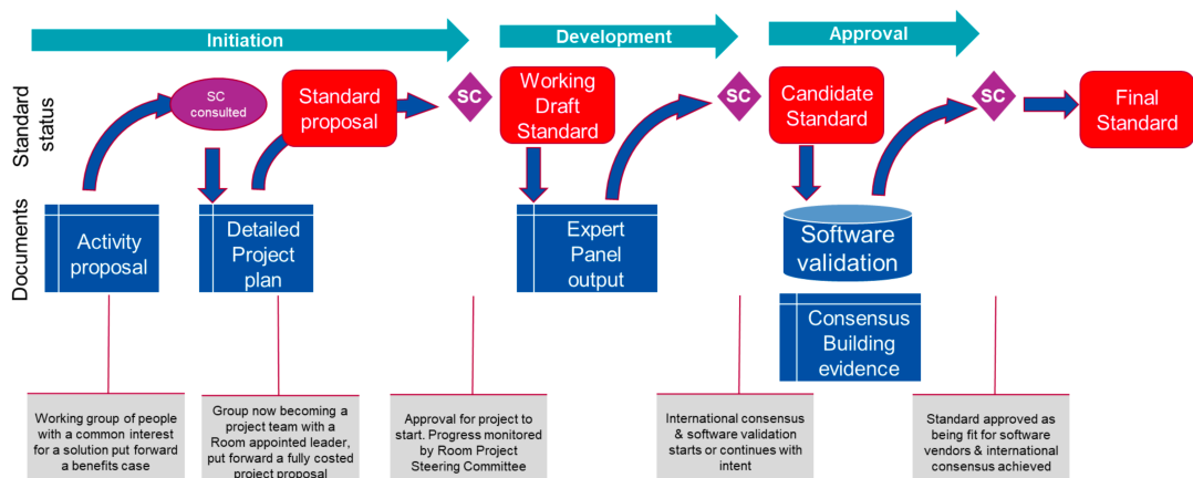
Abb. 3.12: Standardisierungsprozess IFC
