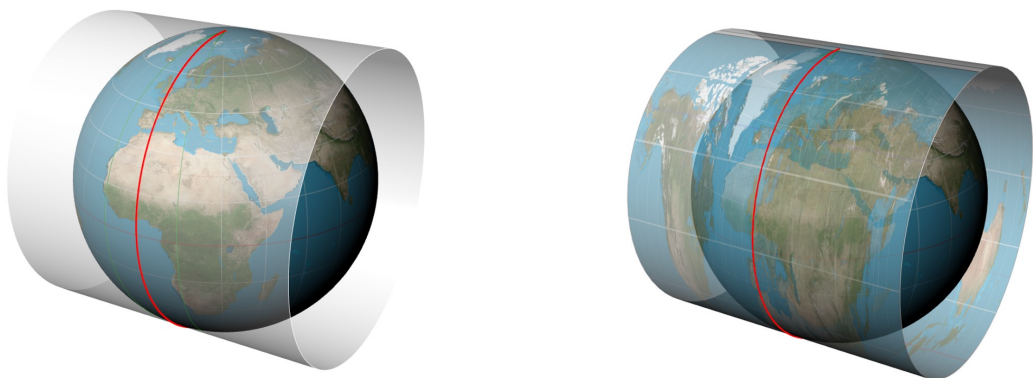
Abb. 3.70: Transversale Mercator-Projektion: transversaler Zylinder (links) und transversale Projektion (rechts)
