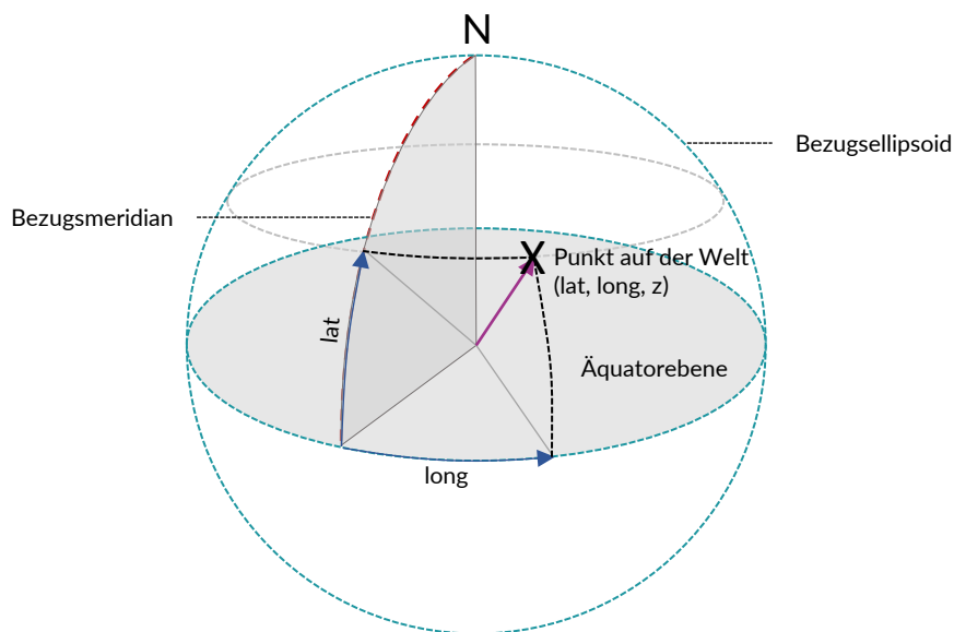
Abb. 3.68: Lagebestimmung mit Polarkoordinaten
