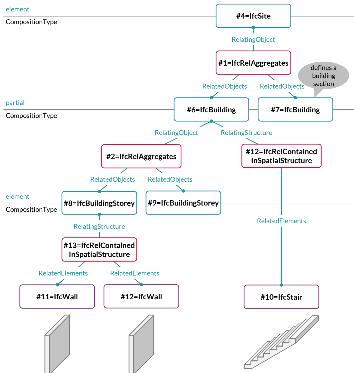
Abb. 3.28: Räumliche Beziehung im Hochbau (IfcRelContainedInSpatialStructure)
