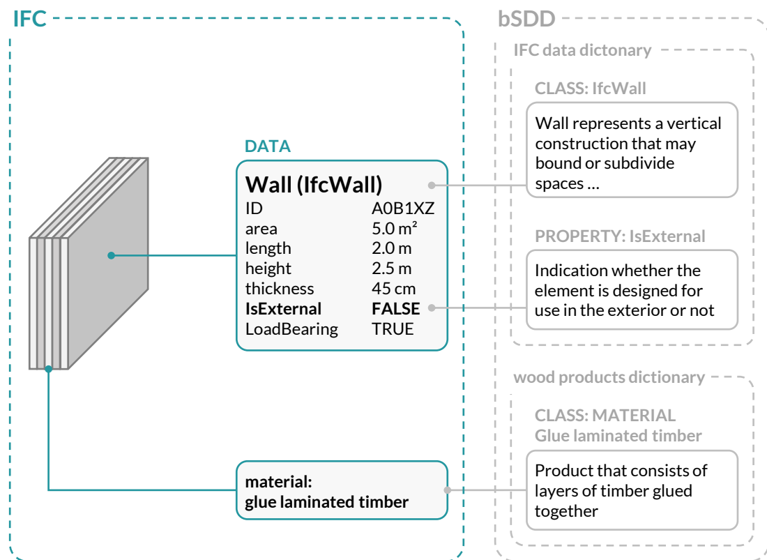
Abb. 3.56: Beispielwand mit Begriffen aus dem bSDD und deren Definitionen
