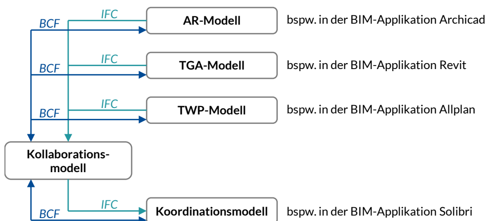
Abb. 3.42: Datenaustausch zwischen den Modellen
