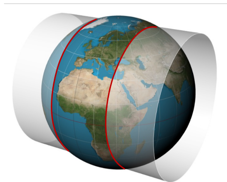
Abb. 3.72: UTM-Projektion mit zwei Berührungsmeridianen
