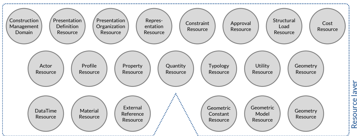
Abb. 3.14: Ressource Layer
