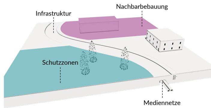
Abb. 3.67: Geographischer Kontext
