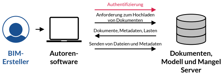
Abb. 3.43: CDE-Kommunikation BIM-Ersteller
